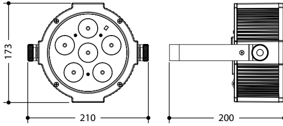
Disegno tecnico
