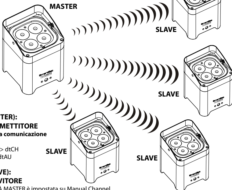
Fig.8 - Configurazione modalità Master/Slave
